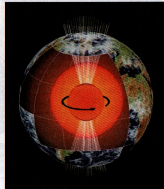
Fig. 11 - Le vrai soleil est dans la Terre. Le noyau a une très haute température et tournait sur lui-même plus vite que la croûte. Leurs spins n'étaient pas alignés l'un sur l'autre. Le récent tremblement de terre du 26/12/04 a pu provoquer un alignement partiel des spins et peut être le premier d'une série d'autres séismes, qui dévoilera les mondes de Gaïa et le vrai Soleil en Son centre. La cause est la Force, la Vie Eternelle, qui fait évoluer tous les corps.
