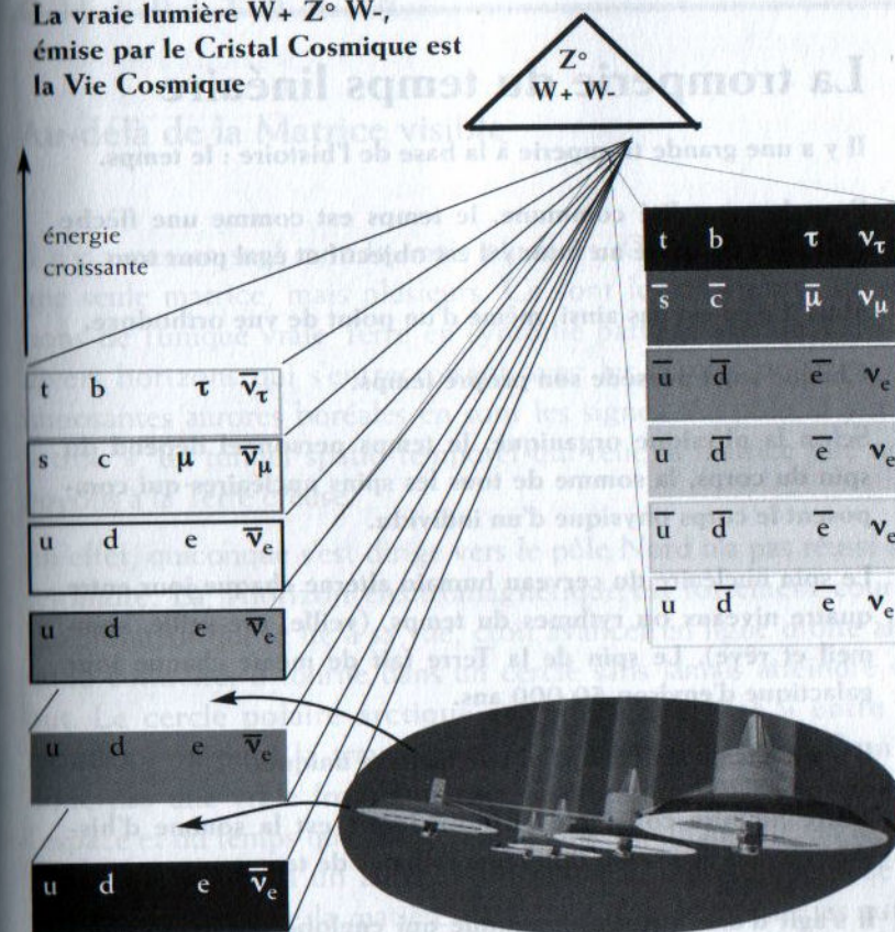
Fig. 26 - Les mondes virtuels sont composés de particules (12+3) reconnues par le Modèle Standard (page xvi) constituant les 4 ELEMENTS. Les 12 premières composent les matrices ou réalités virtuelles incluant les corps virtuels de l'homme. Celui d'un « mort » est constitué d'AIR, celui d'un « vivant » est constitué de TERRE. Ces deux corps sont animés en alternance quand le corps de lumière, le véritable Soi fusionne avec l'un d'eux. A chaque ELEMENT de matière, correspond un anti-ELEMENT constitué d'anti-matière. Les corps et les anti-corps ne peuvent pas se rencontrer mais la fusion intérieure est possible en éliminant la dualité et en retrouvant l'amour de soi. Le Cristal cosmique célèbre le mariage alchimique entre les corps éphémères et le corps de Lumière éternel.
