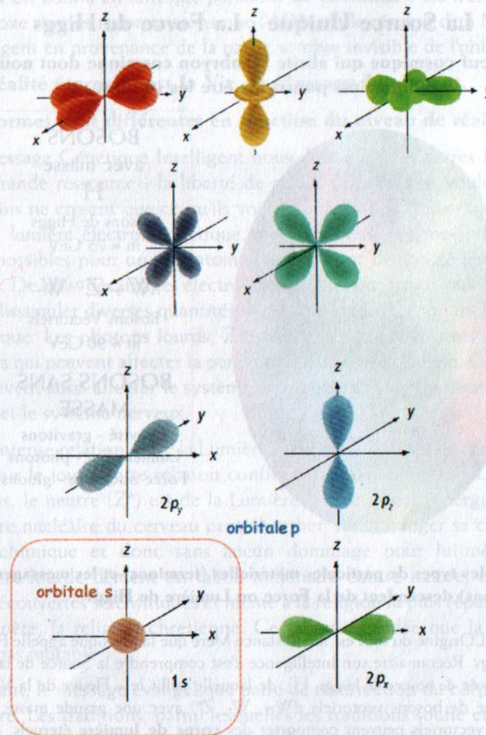
Fig. 7 - Les formes d'un atome dépendent du niveau d'énergie qu'atteignent les électrons selon leur interaction avec des photons ordinaires, des messagers de lumière électromagnétique ou des quanta. Cette interaction n'est pas aléatoire mais causée par la relation entre la matière et les forces GEN. Seul le niveau d'énergie minimum (1s) présente une forme sphérique.
