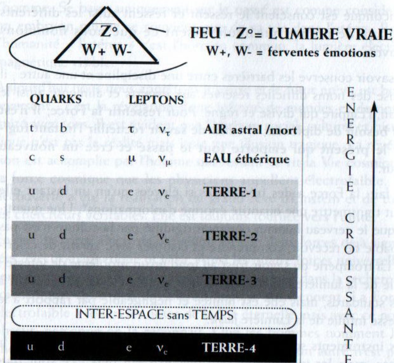
Fig. 23 - Le FEU cosmique est le message génétique qui informe, c'est-à-dire qui génère les formes composées des trois différents types de matière, celles que les anciens nommèrent AIR, EAU et TERRE. Le modèle standard de la physique reconnaît une structure analogue, c'est-à-dire trois types de matière, composée chacune de 4 particules élémentaires, au total 12, toutes liées au FEU ( W^+ , Z^0 , W^- ). L'élément TERRE est un état lié par des forces contraignantes (la gravité et la force nucléaire forte), donc « subdivisé » sur des bandes d'énergies, séparées entre elles par un gap. TERRE 1, 2, 3, 4, sont les 4 phases nucléaires, ou Saisons, entre lesquelles, la planète a alterné jusqu'à présent, et entre lesquelles le cerveau humain alterne toujours. Celle que nous vivons aujourd'hui est la TERRE 4, l'Hiver nucléaire qui a duré treize mille ans, l'état le plus pauvre en énergie vitale, correspondant à l'état de veille. Les gaps entre les phases les plus froides et les phases supérieures sont les inter-espaces sans temps, cachés par le « voile » ou le champ électromagnétique. C'est ce que nous vivons comme oublié et où sont créées les interférences électromagnétiques.
