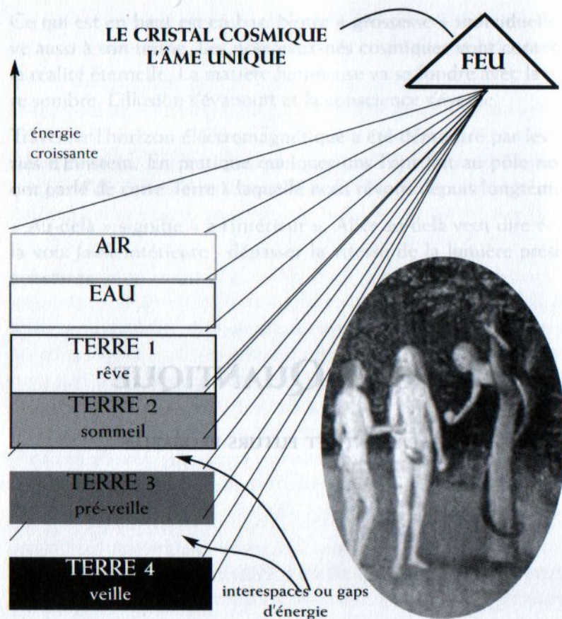
Fig. 25 - La « chute » de l'homme se réfère au spin des particules nucléaires qui composent le corps physique. L'élément TERRE est un état limité et possède des bandes d'énergies séparées par des gaps. Le cerveau humain alterne chaque jour sur ces quatre phases (les états de veille, pré-veille, sommeil et rêve) mais « oublie » et considère l'état de veille comme la seule réalité. Les gaps correspondent au subconscient généralement dominé par l'Empire, un état de séparation. Les entités coincées dans les interespaces peuvent interférer avec le cerveau humain si les terriens acceptent. Ces transmissions sont étrangères à la Vie. Les terriens qui acceptent, perdent le contact avec leur âme, leur vraie identité. Ils oublient alors la compassion et l'amour, le rêve d'un monde plus sain et plus juste ; ils répriment leurs émotions et ont en échange privilèges et pouvoir dans le monde de la surface de la Terre.
