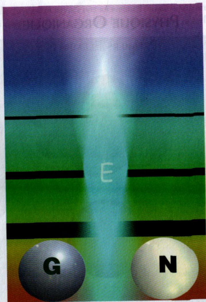
Fig. 2 - Il existe aussi différents types de lumière. Les trois forces, GEN (Gravité, Electro-faible, Nucléaire) ont leurs propres messagers. La Force électrofaible est la seule qui n'est pas limitée au seul niveau visible et qui a deux faces, l'une obscure, l'autre lumineuse. La face obscure de la Force est la lumière électromagnétique trompeuse. La face lumineuse est la lumière cristalline, que la Physique nomme faible ; elle a les mêmes messagers que la Force ( W^+ , Z^0 , W^- ), elle relie différents types de matière et elle viole la parité droite-gauche. © élaboré par G.C.
