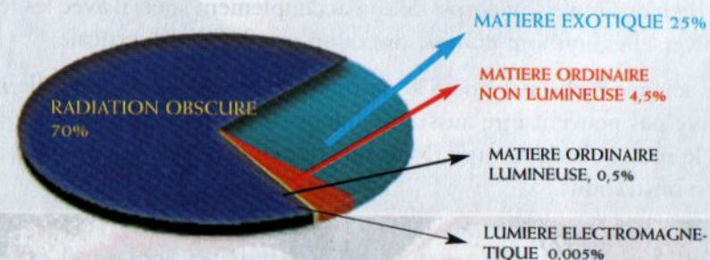
Fig. 3 - La matière lumineuse n'est pas l'unique type de matière, mais la seule qui émet, absorbe et reflète la lumière électromagnétique. Cette lumière est le « voile » de l'illusion qui cache la vraie lumière obscure, les 70% du tout considérables, qui génèrent une infinité d'univers vivants, intelligents et conscients de l'unité organique.
