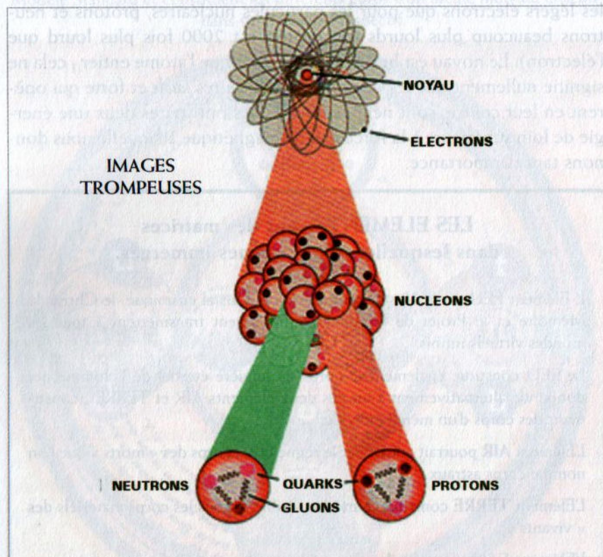
Fig. 10 - Cette représentation de l'atome est courante pourtant elle contient une série de tromperies : (a) les électrons ne sont pas de petites balles mais des nuages électroniques (b) les quarks sont bien plus petits que les gluons et sont en fait des mini-trous de l'espace temps (c) les bosons vectoriels ( W^+ , W^- , Z^0 ), messagers de la Force nucléaire faible , ne sont pas présents, tandis que les gluons, messagers de la Force nucléaire forte, oui. La Force nucléaire faible est toujours négligée parce que son rayon d'action est petit ( 10^{-16} cm) pourtant son énergie est grande.
