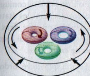
Fig. 15 - Images intuitives des trois quarks qui composent une particule nucléaire (protons et neutrons). L'Anneau est là si la rotation est basse ; il n'y est pas si elle est élevée.
