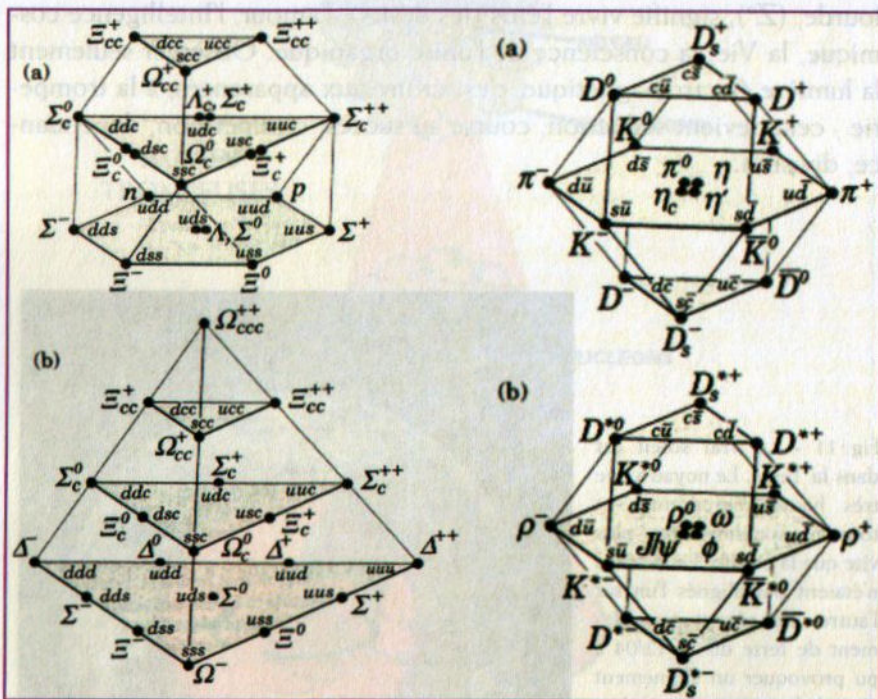
Fig. 12 - Les états Supersymétriques démontrent le lien intime entre les quarks u e d, qui composent le noyau de l'atome, et les particules qui composent la masse obscure (neutrinos, quarks et beaucoup d'autres).
